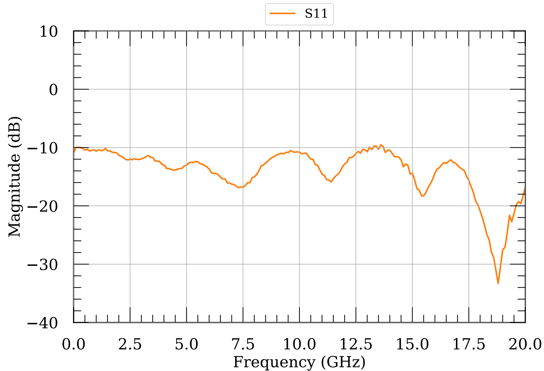
LNA S-params module051
